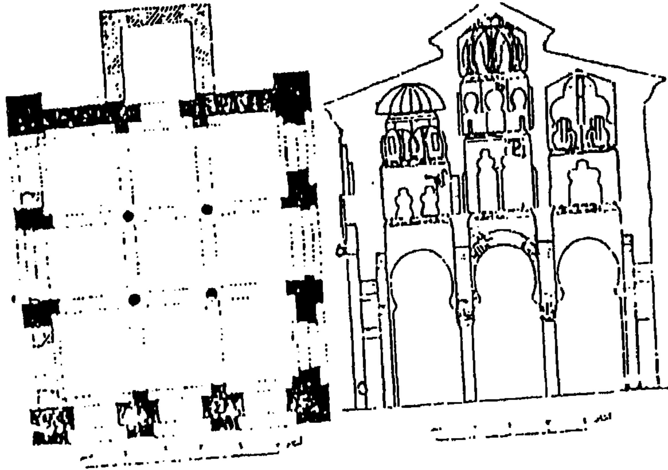
الشكل رقم (٢٩) مسقط أفقي وقطاع رأسي لمسجد الباب المردوم ببليظة (عن : Moreno)
