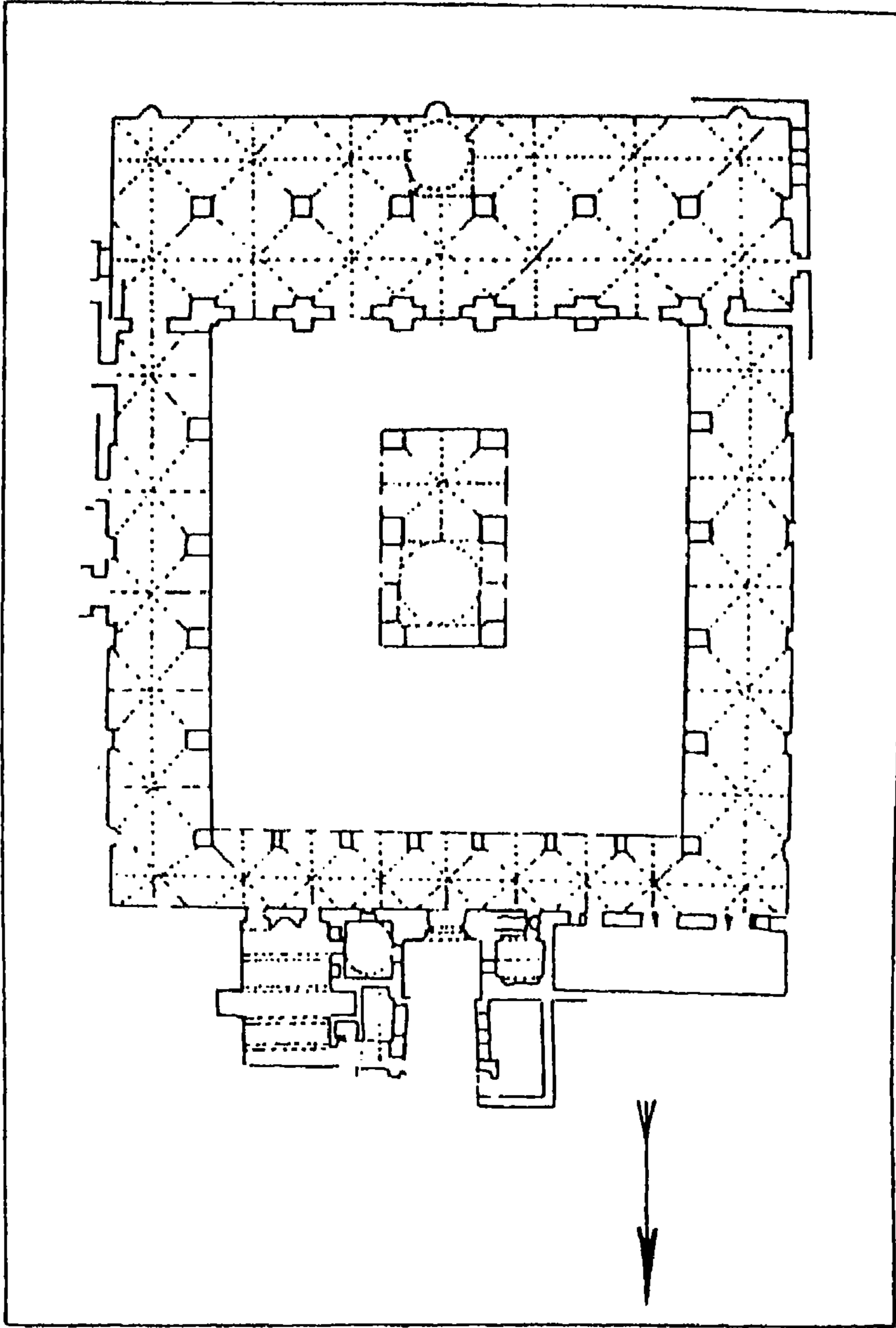
الشكل رقم (١٨) مسقط أفقي للجامع المنصوري الكبير بطرابلس الشام ببلنات (عن : Liebich)
