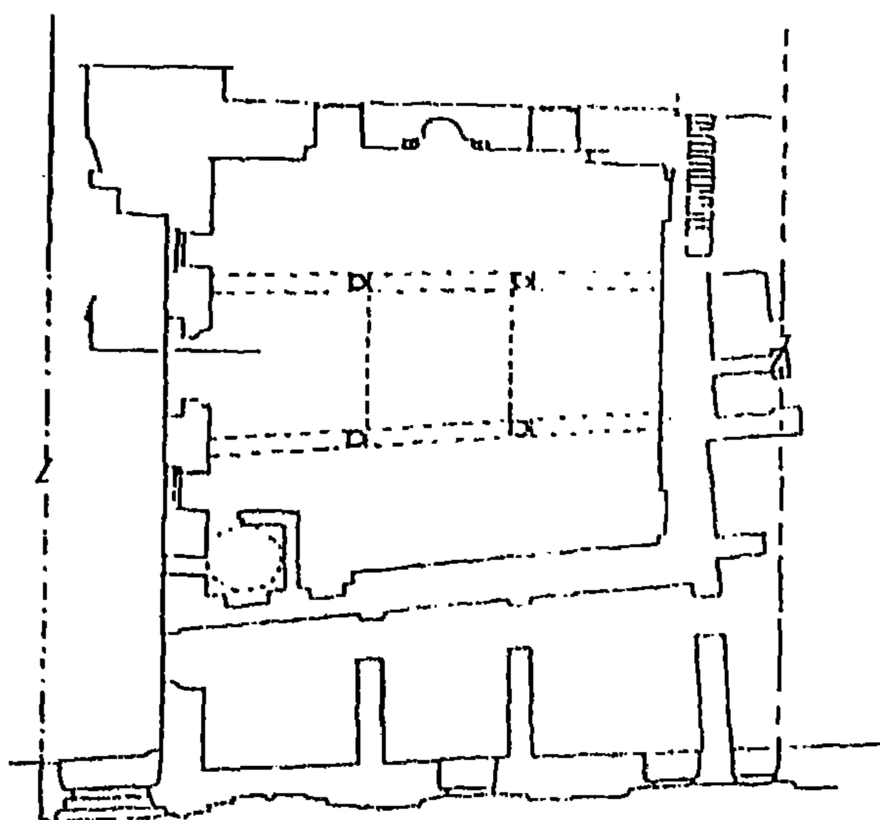
الشكل رقم (٢٤) مكرر) مسقط أفقي للمدرسة الطبرسية بالأزهر بالقاهرة (عن المجلس الأعلى للآثار)
